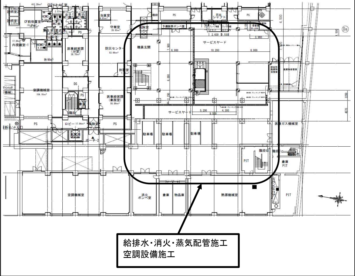
平面図
